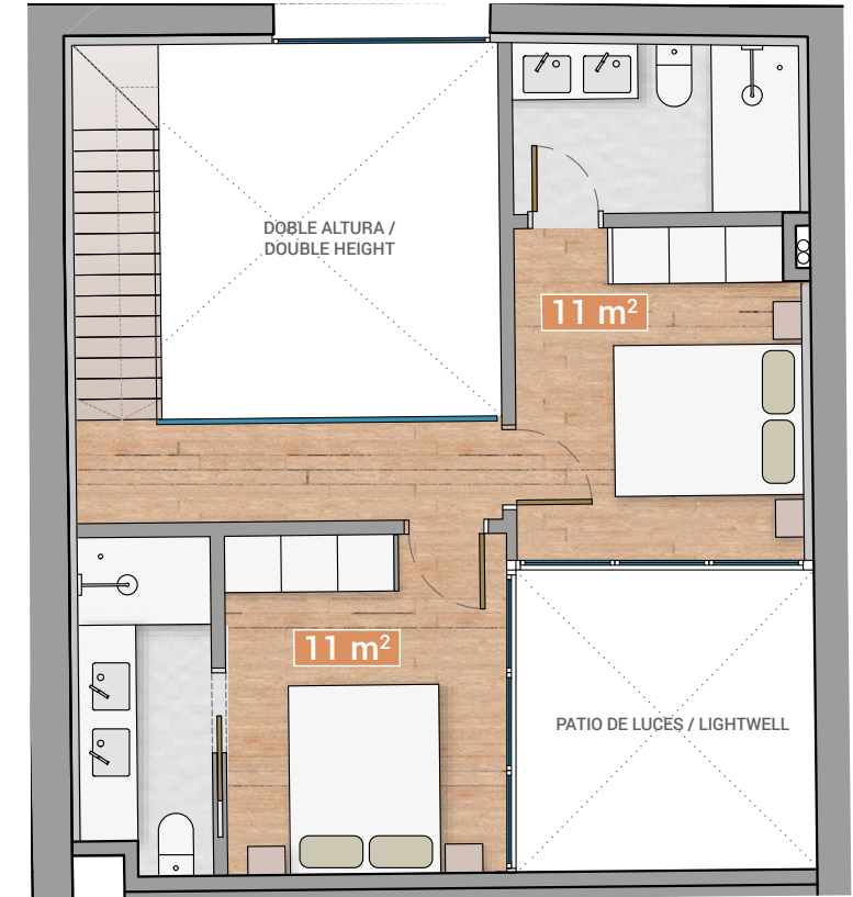
PLANTA PRIMERA / FIRST FLOOR
